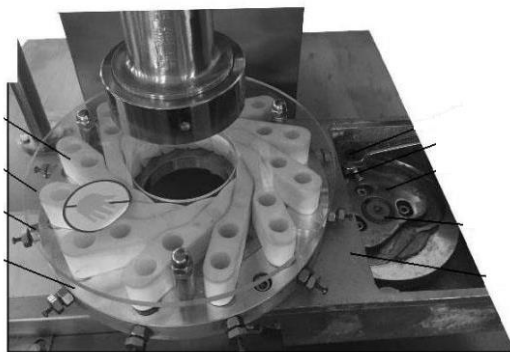
Рис.9 Узел формирования заготовок.
