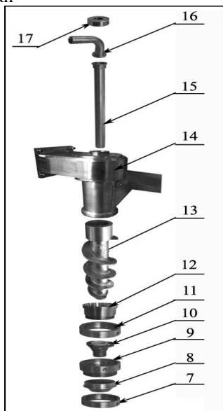
Рис.2 Основные элементы подачи теста (формирование тестовой трубы)
