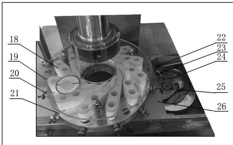
Рис.4 Формирователь, основные элементы
